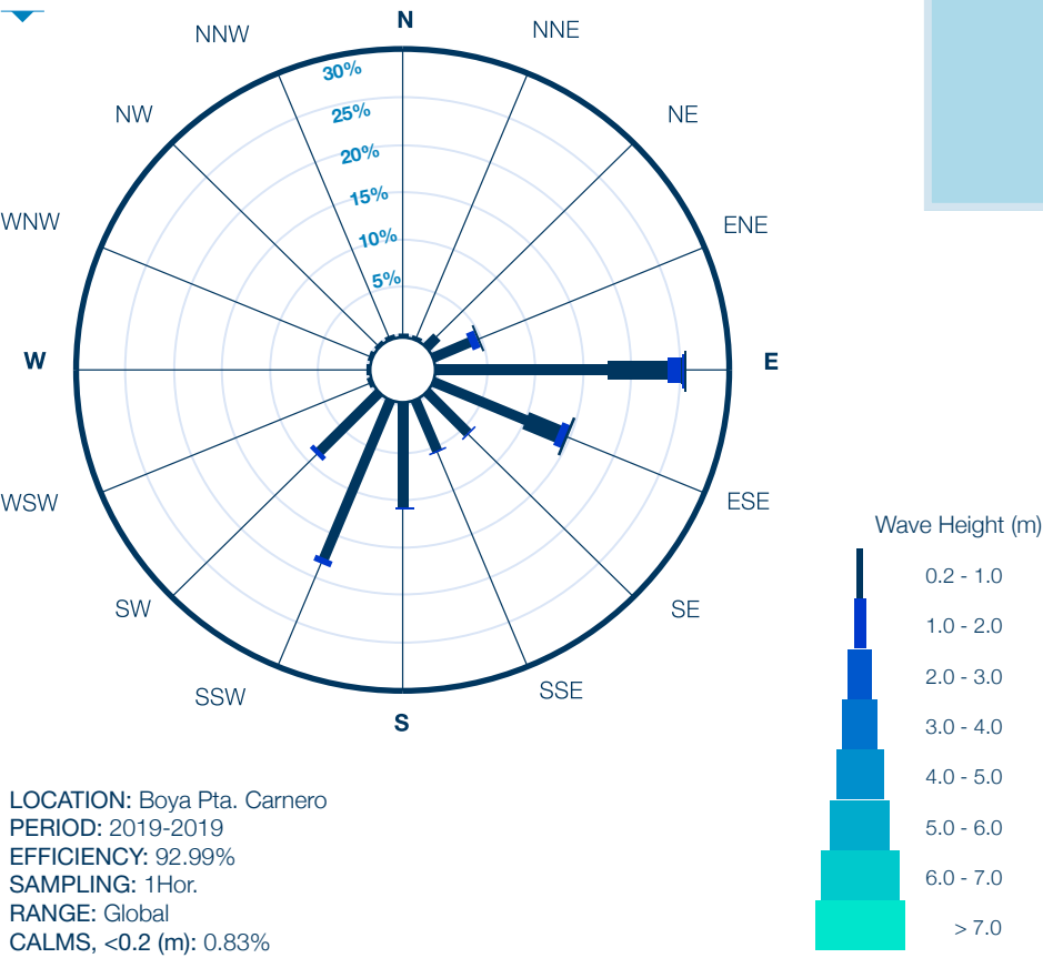
FIG 2: WAVE ROSE Buoy Algeciras - Punta Carnero
